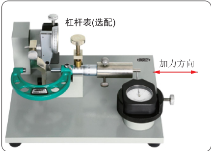
测量千分尺测微螺杆的轴向窜动
