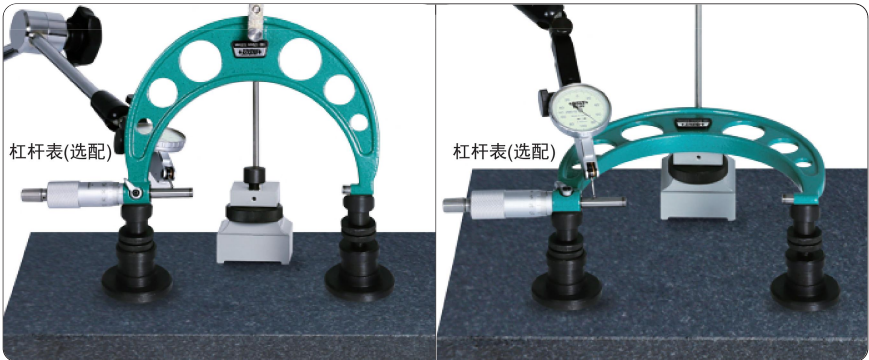
测量千分尺测砧与测微螺杆测量面的相对偏移
