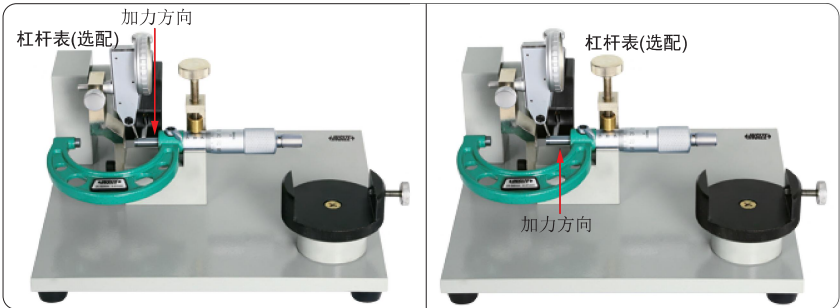
测量千分尺测微螺杆的径向摆动
